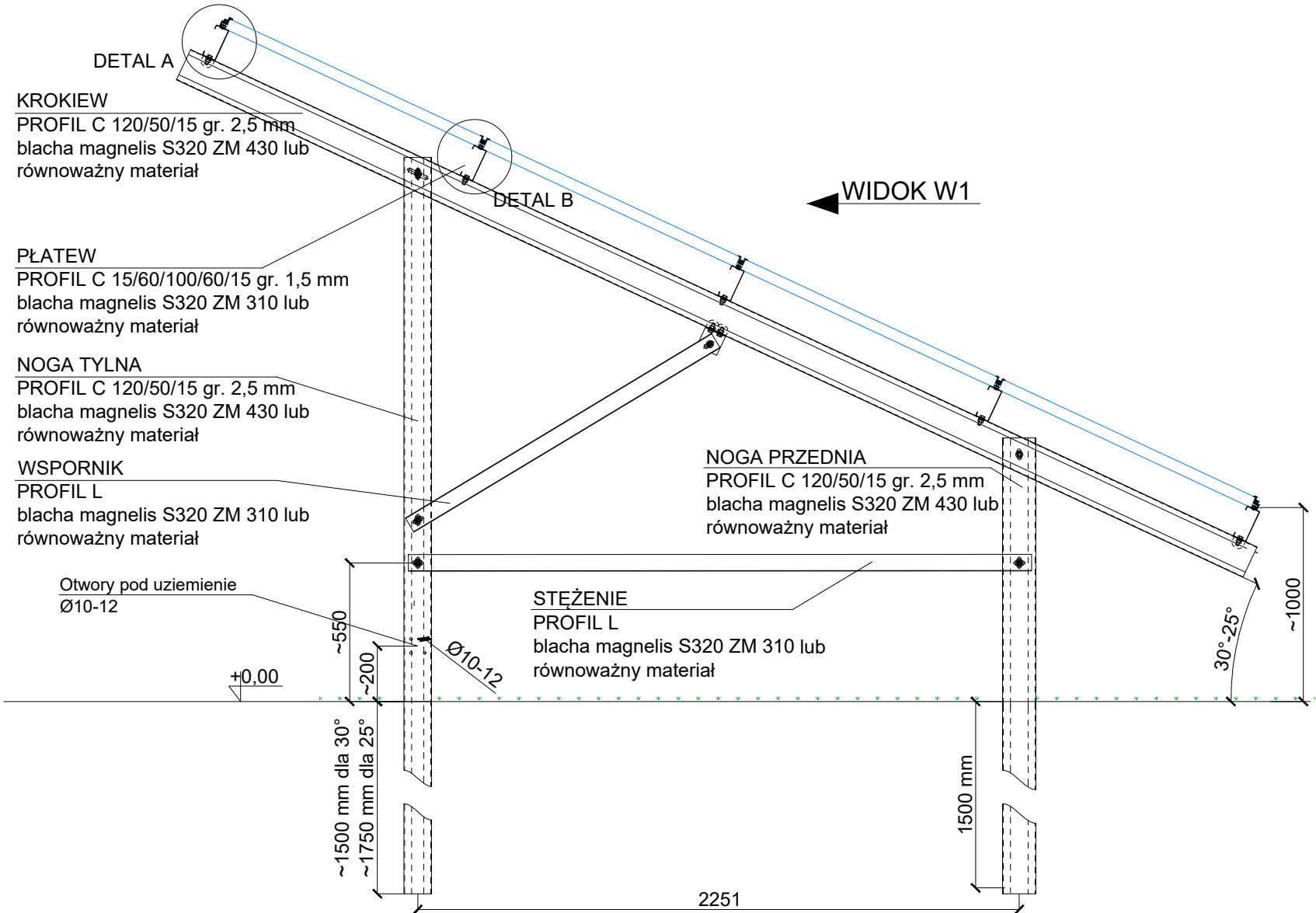
PRZEKRÓJ A-A
